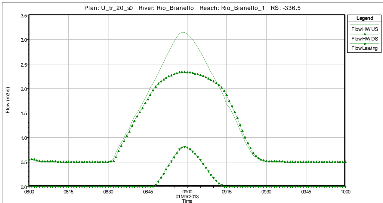
Figura 12: Idrogrammi relativi alla Lateral Structure a monte del tratto tombato per Tr = 20 anni nello stato di progetto.
