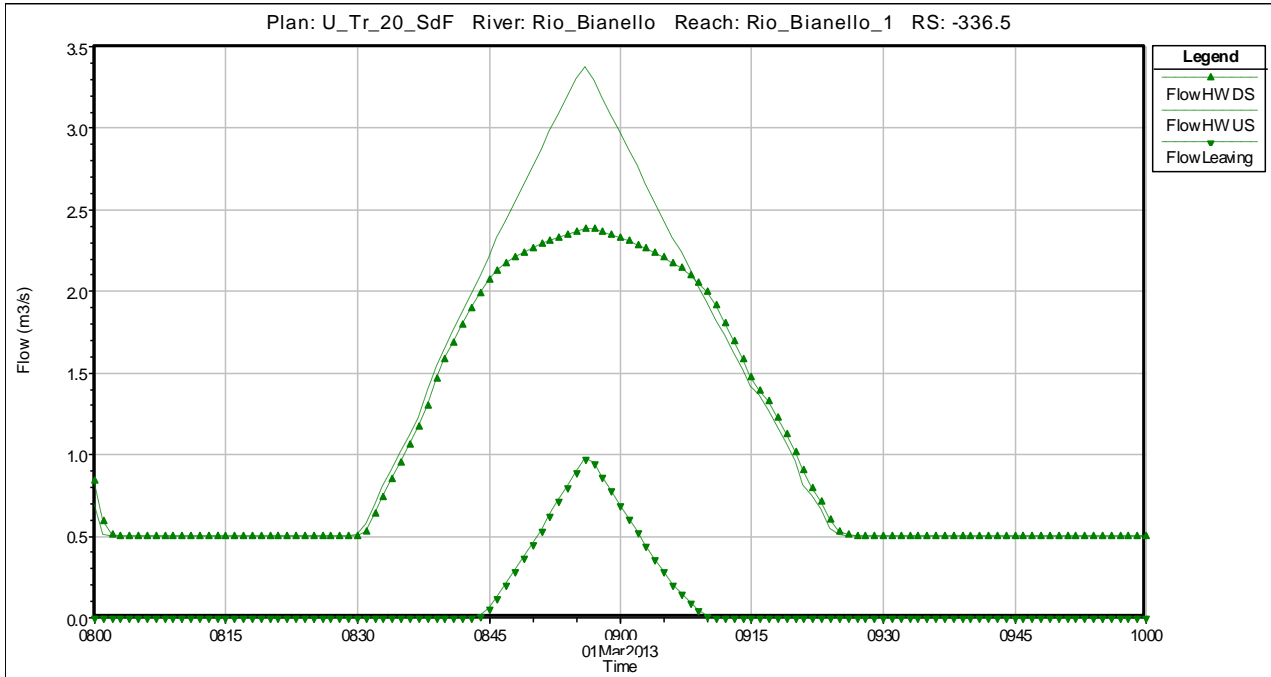
Figura 7: Idrogrammi relativi alla Lateral Structure a monte del tratto tombato (tra le sezioni 3 e 4) per Tr = 20 anni nello stato di fatto.
