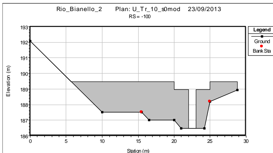
Figura 11: Creazione della briglia aperta sulla sezione 2.
