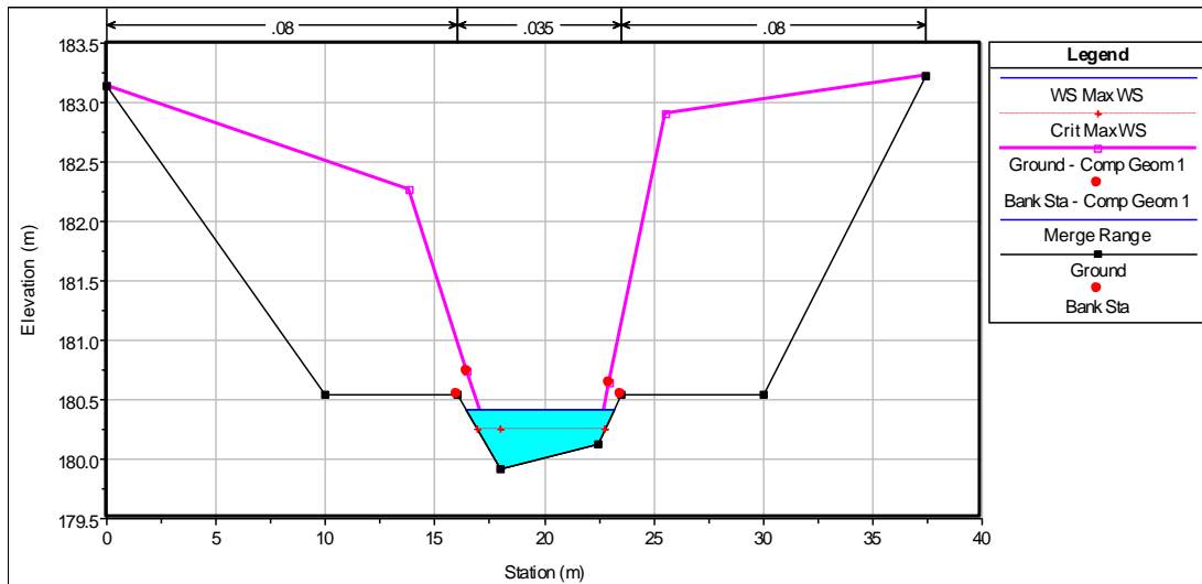
Figura 10: Confronto tra la sezione a monte del ponticello che conduce al castello di Bianello, rappresentata nello stato di fatto e nello stato di progetto a seguito degli allargamenti previsti.
