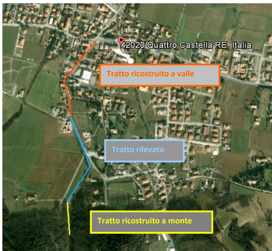
Figura 1: Estensione dei tratti rilevati e simulati.
