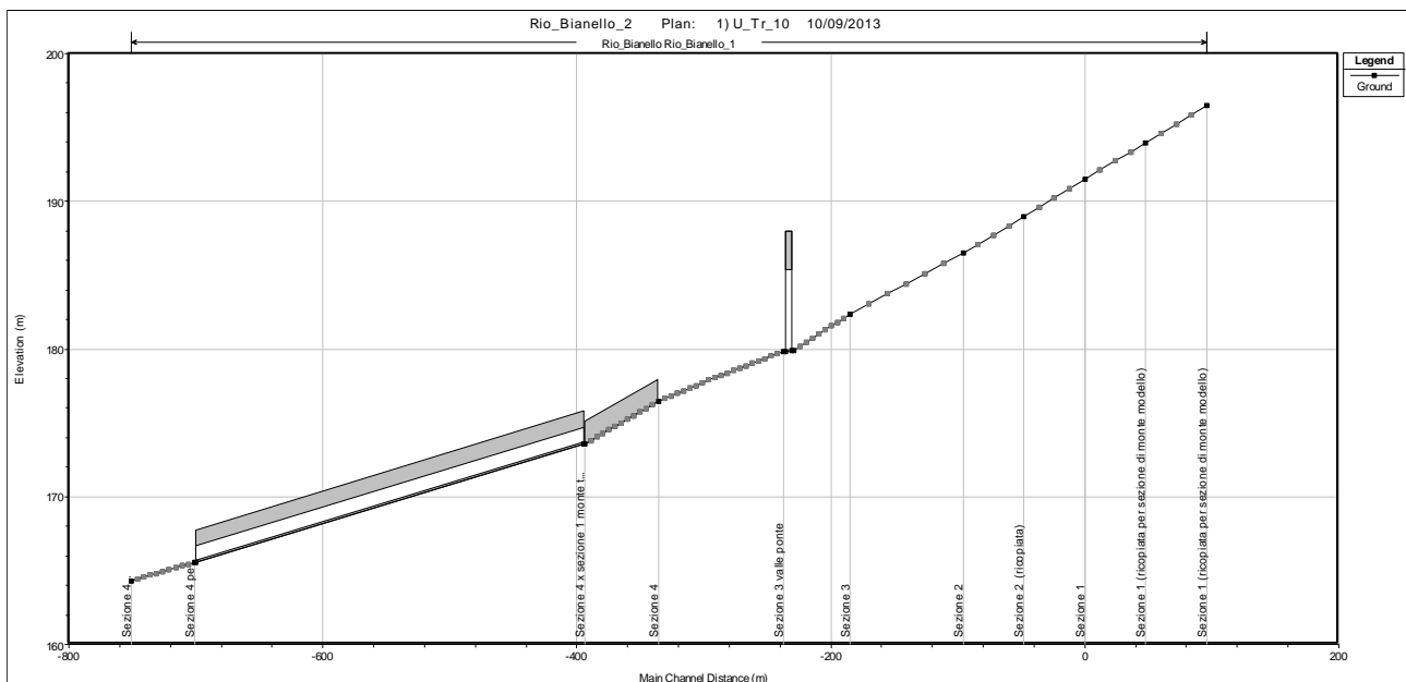
Figura 2: Profilo longitudinale del Rio Bianello nello stato di fatto.
