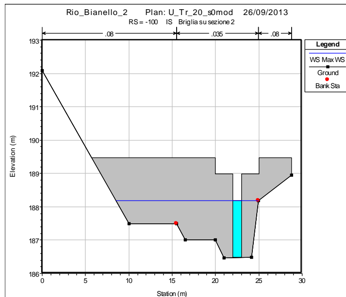
Figura 14: Briglia su sezione 2 Tr = 20 anni nello stato di progetto.
