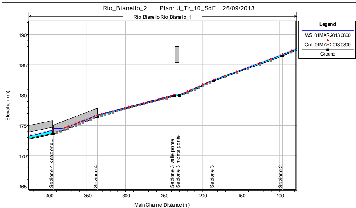
Figura 6: Esempio del profilo del pelo libero per Q = 0.5 \text{ m}^3/\text{s} .
