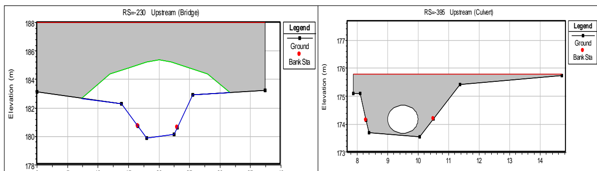
Figura 3: a sinistra schematizzazione del ponticello che conduce al castello; a destra schematizzazione dell'imbocco del tratto tombato.
