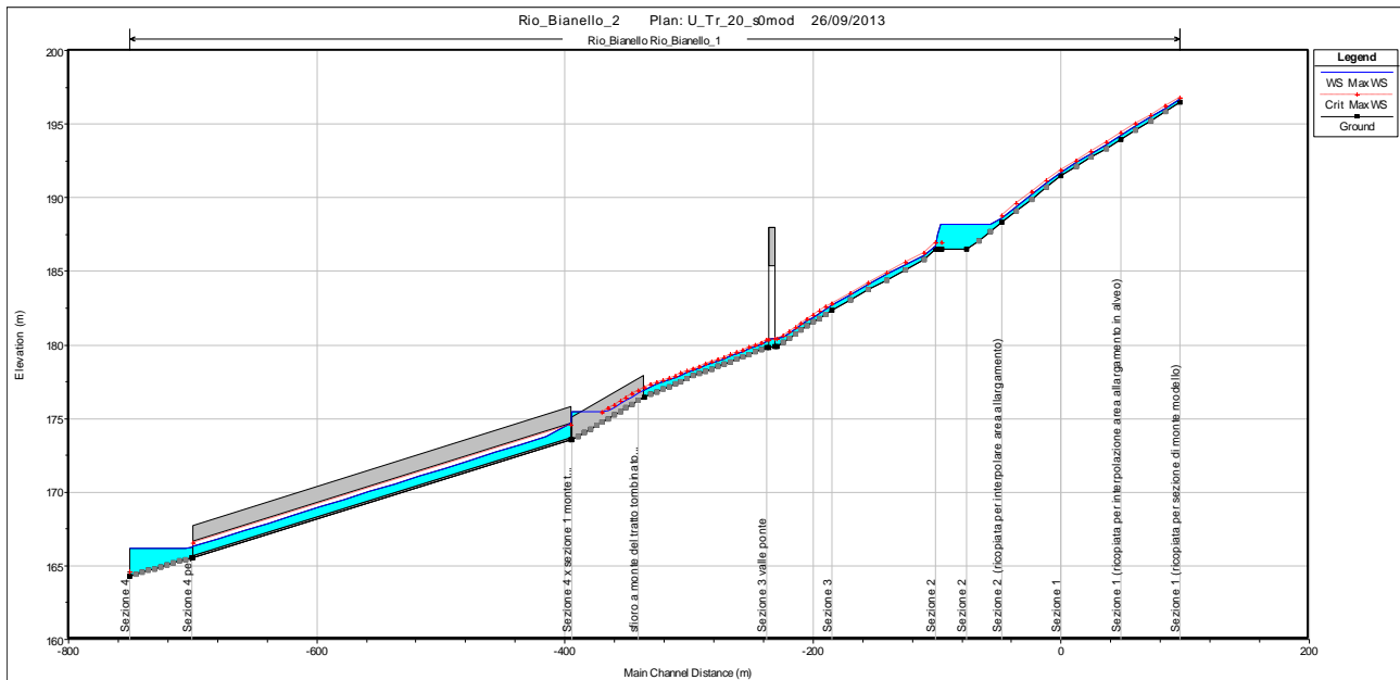
Figura 13: Profilo del pelo libero per Tr = 20 anni nello stato di progetto. Si noti l'effetto della briglia aperta nel tratto di monte
