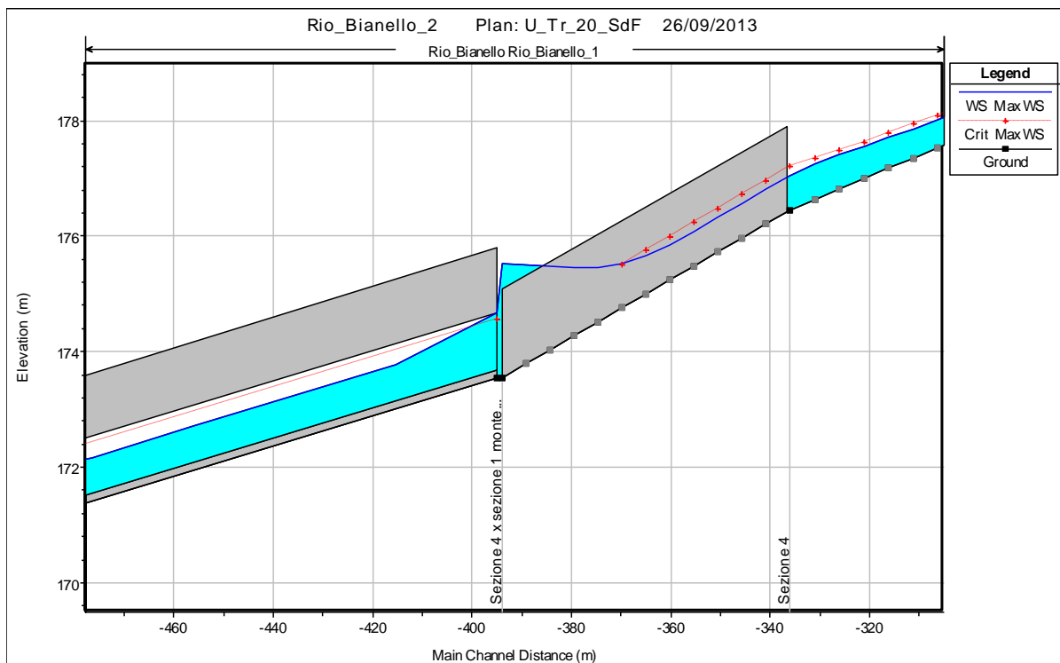
Figura 8: Dettaglio del tratto tombato con la schematizzazione della Lateral Structure.
