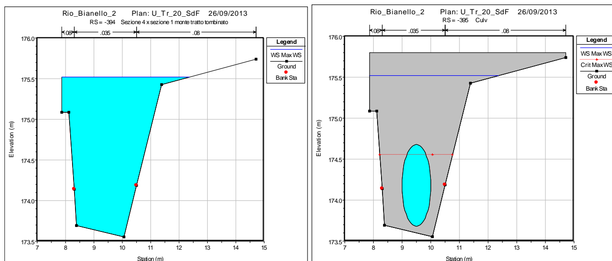
Figura 9: Quota del pelo libero nella sezione 4 a monte del tratto tombato.
